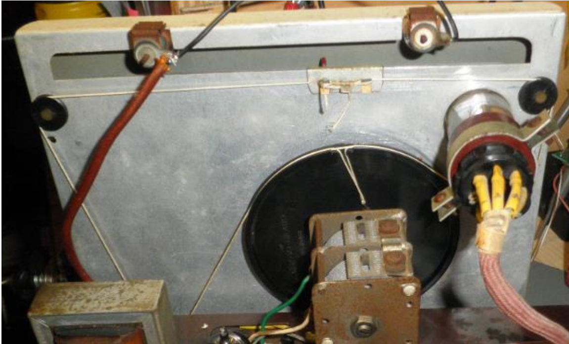
Figura 2, Cordicella di sintonia sostituita
